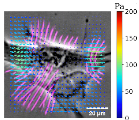
図 2. 機械学習によるシワ・収縮力変換
